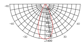
Chóa crom đen
