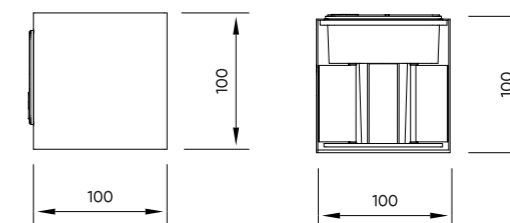
Kích thước
